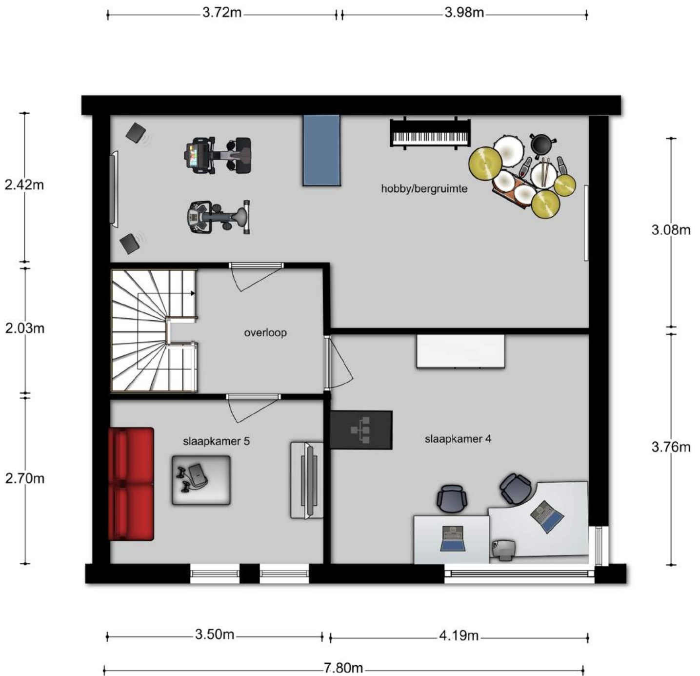
TWEEDE VERDIEPING 3-6
